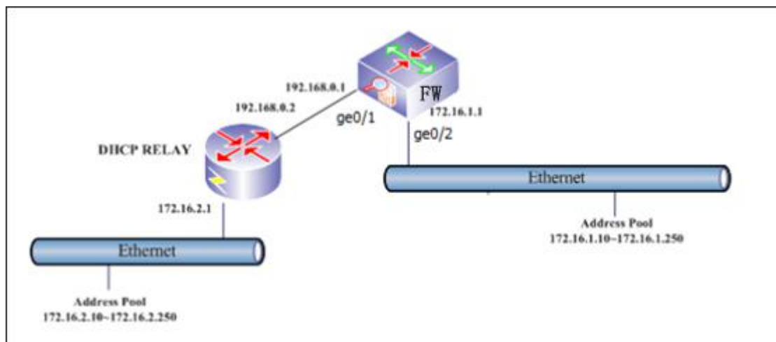
图 17-1 DHCP 服务配置案例组网图
