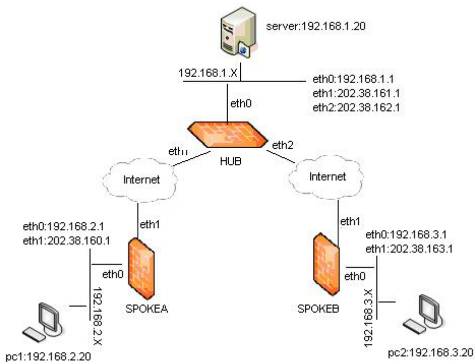
图 29-2 案例组网图
