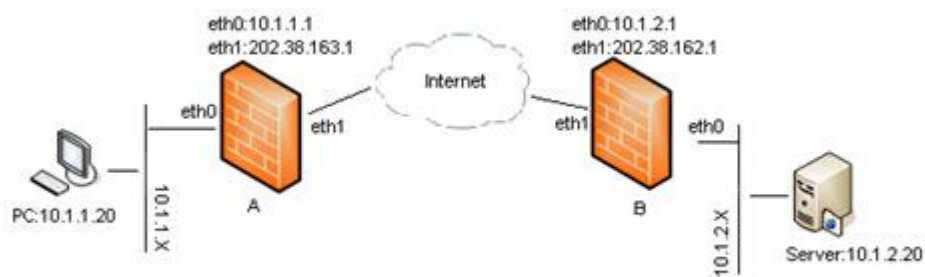
图 29-1 案例组网图
