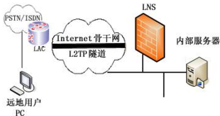
拨号用户通过 LAC 远程接入 LNS
