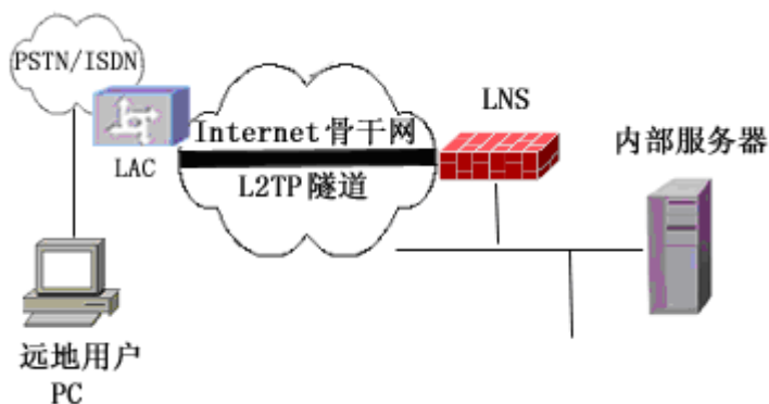
(2) 拨号用户通过 LAC 远程接入 LNS
