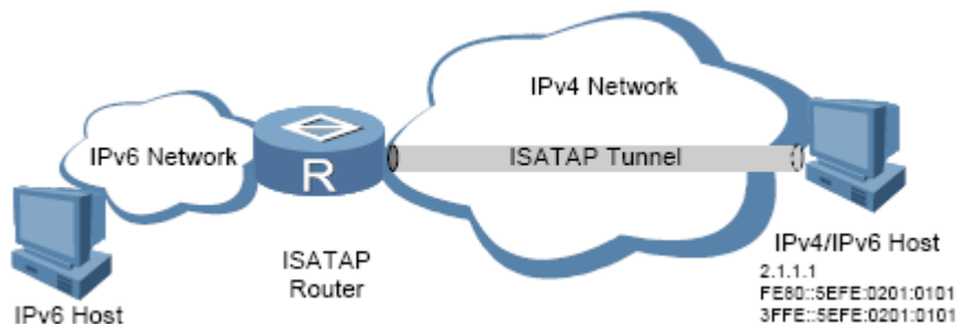
图 7-8 ISATAP 隧道
