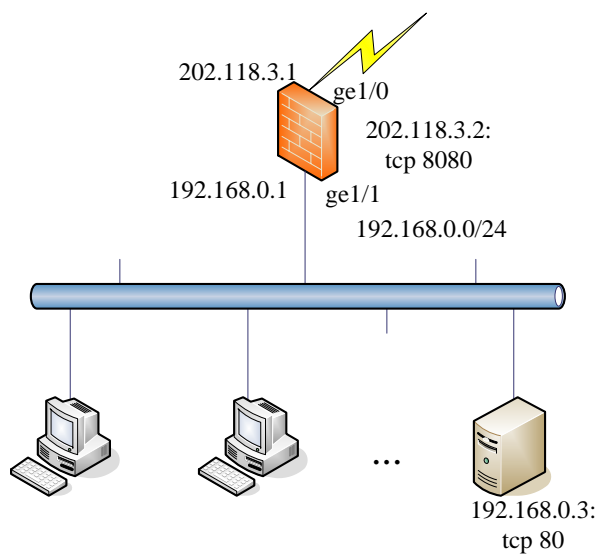
图 15-3 配置 destination NAT 案例组网图 a
